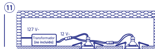
Diagrama para instalar una lámpara a 12 V-
